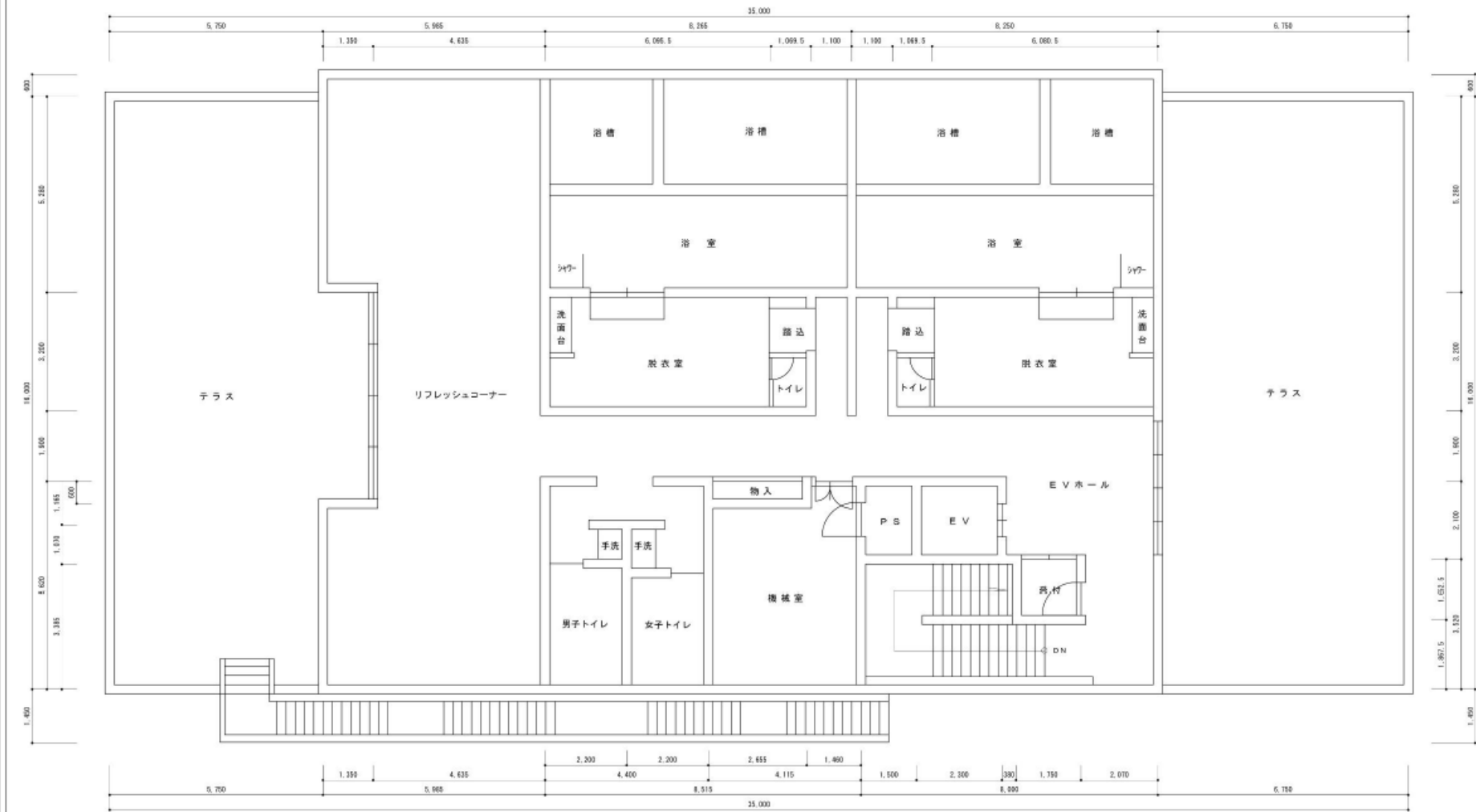
長浜保健センター 3 階平面図 S=1:100
